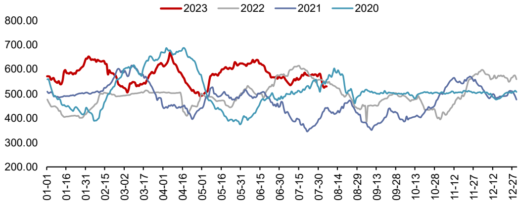
图 11：秦皇岛港煤炭库存（万吨）
