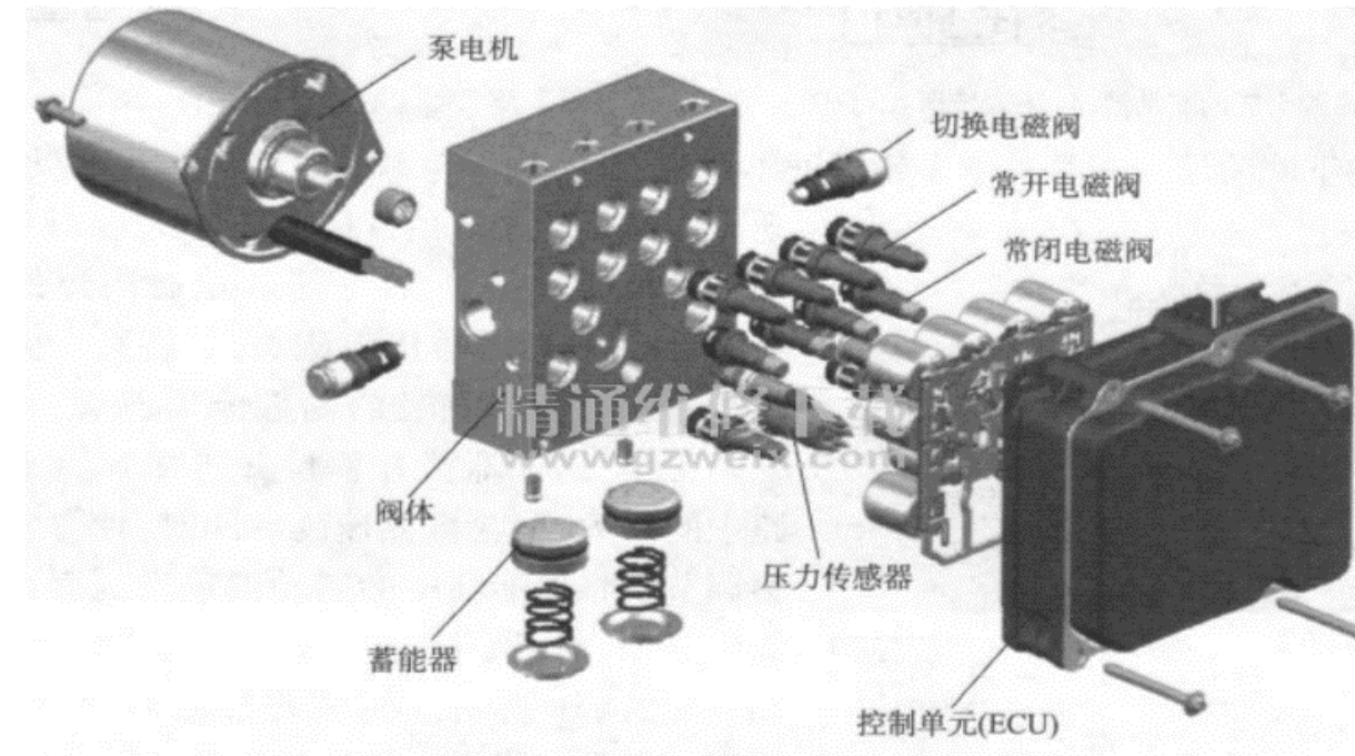
图：ESP产品构成
