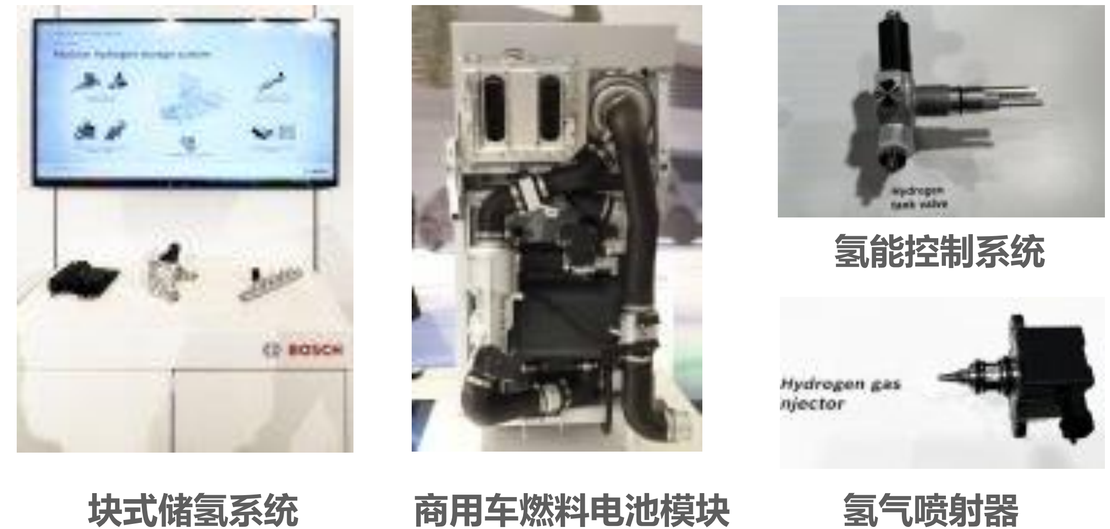
图：博世氢动力系统产品谱系
