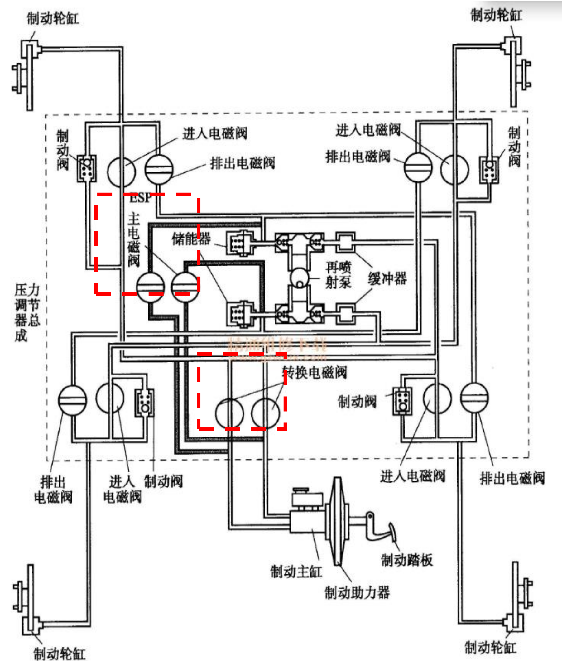
图：博世ESP液压控制单元结构
