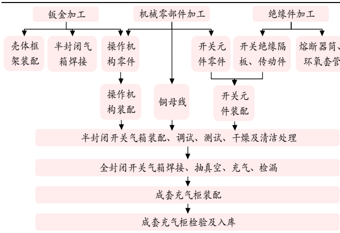
图表 2.C-GIS 生产流程
