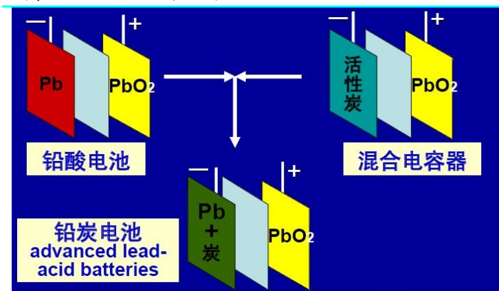
图表1 铅炭电池原理图
