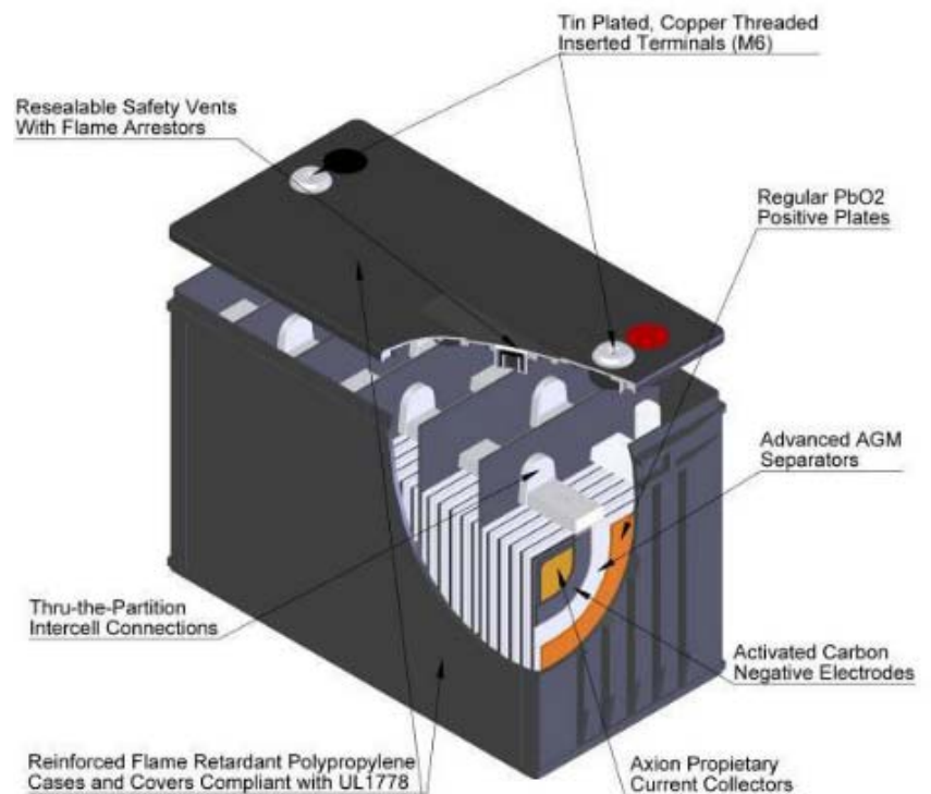
图表 2 铅炭电池结构示意图
