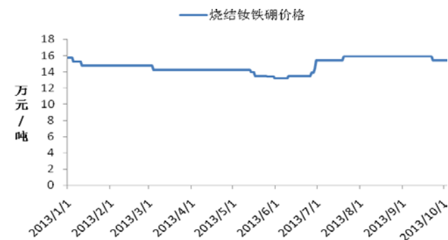
图 2: 2013 年 1-10 月烧结钨铁硼磁材价格
