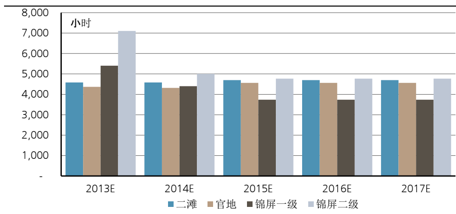
图表 5: 雅砻江下游主要电站利用小时数假设
