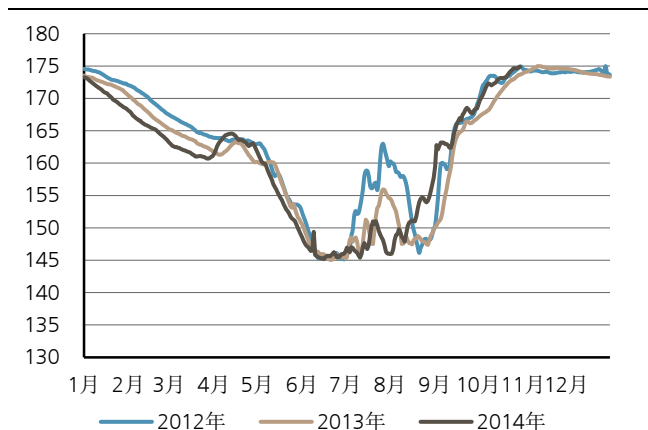
图表 4: 三峡上游水位 (米)
