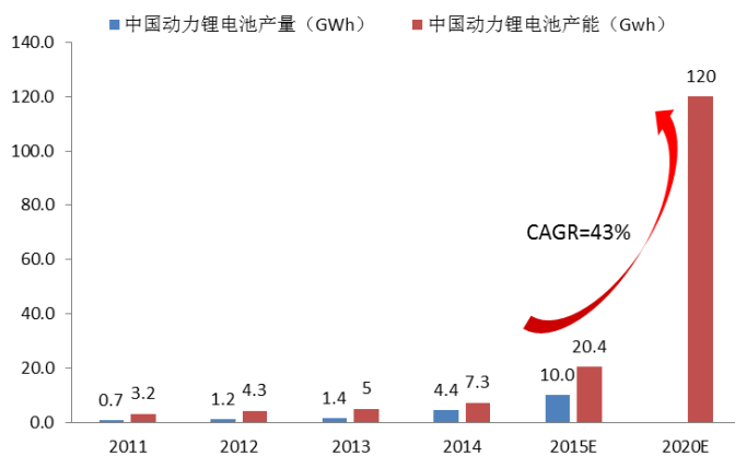
图 2: “十三五”期间我国动力锂电池产能复合增速至少将达到 43%
