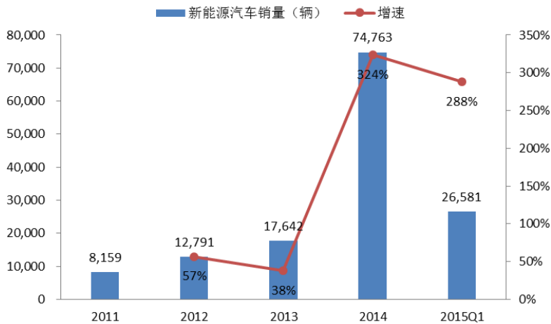
图 1: 2014 年起我国新能源汽车销量进入高速增长阶段
