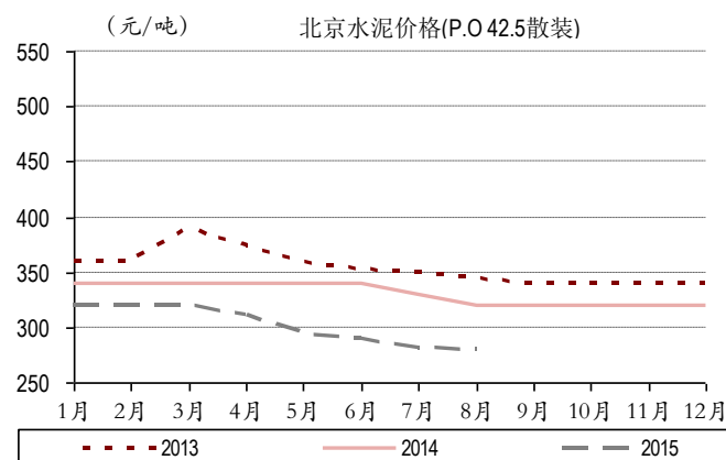
图表 6. 北京地区水泥价格走势
