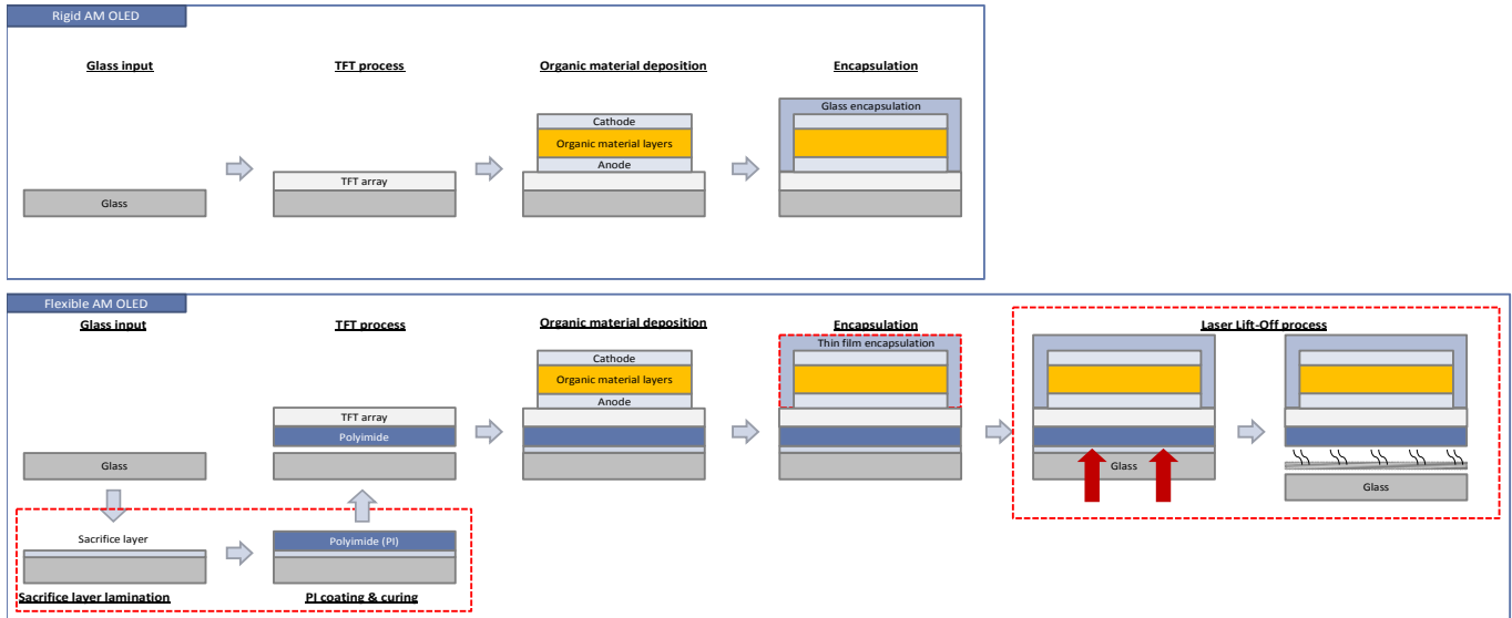
图表 5: 从最初的基板切割、到准分子激光退火和激光维修、再到最后的激光剥离(LLO), 整个 OLED 生产流程处处体现了激光技术的应用
