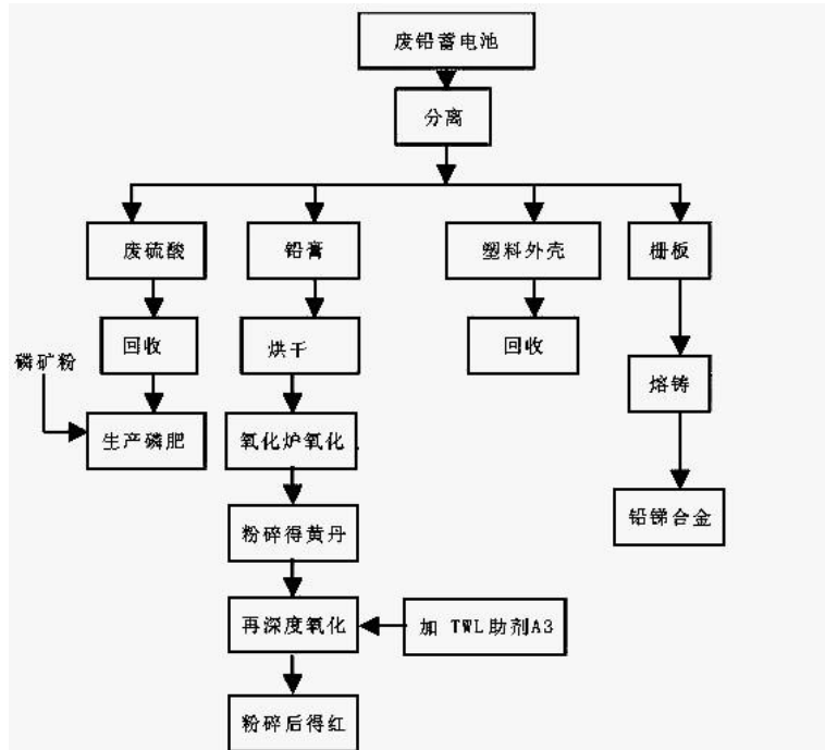
图表 1. 经典废旧铅酸电池回收流程
