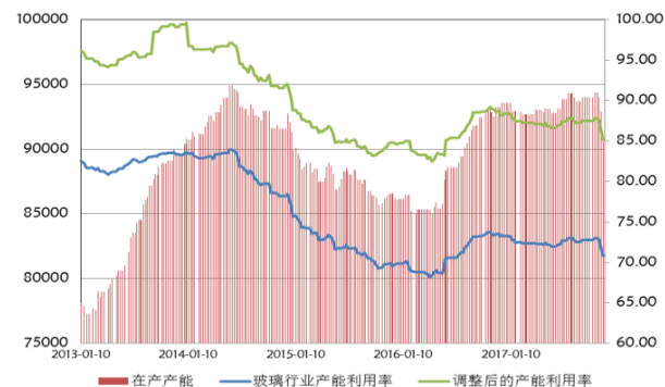
图 16：玻璃在产产能及产能利用率（%）
