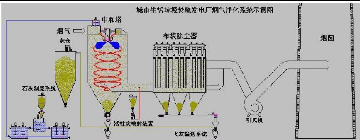
图表 18 垃圾焚烧发电锅炉示意图
