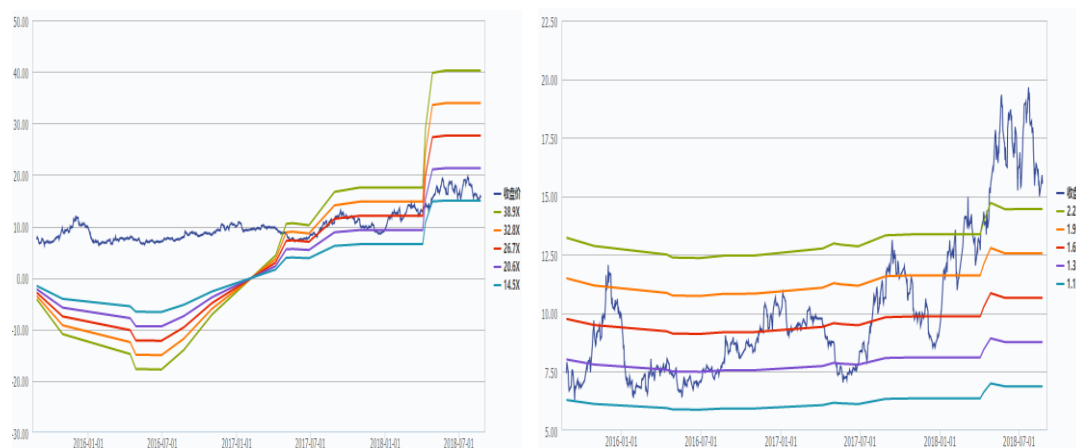
图表 2 新安股份[600596] PE/PB-band
