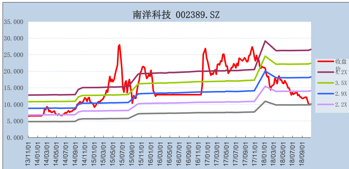
图 2：南洋科技（002389）历史 PB Band
