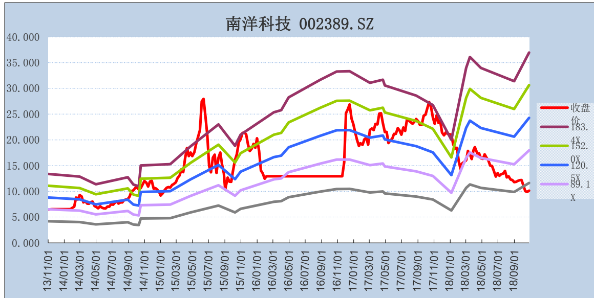
图 1：南洋科技（002389）历史 PE Band
