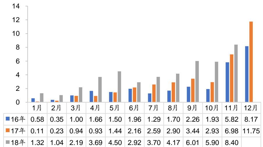
图3: 中国动力电池装机量 (GWh)
