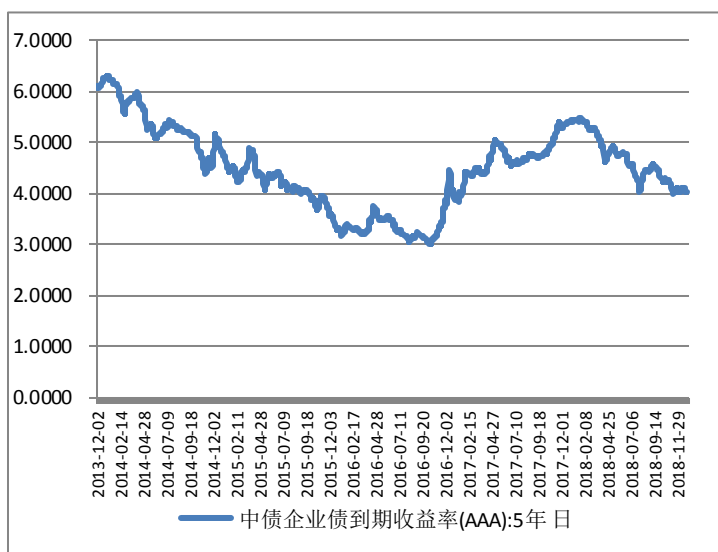
图 3:5 年期 AAA 企业债发行利率变动
