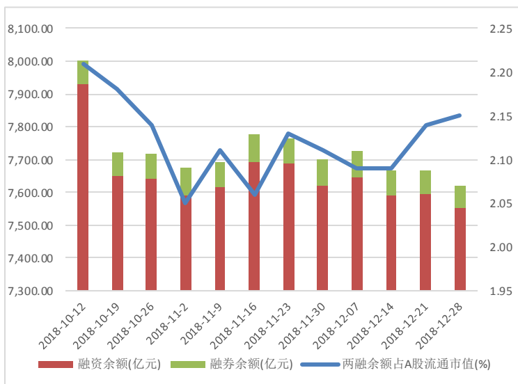
图 2:两融余额变动
