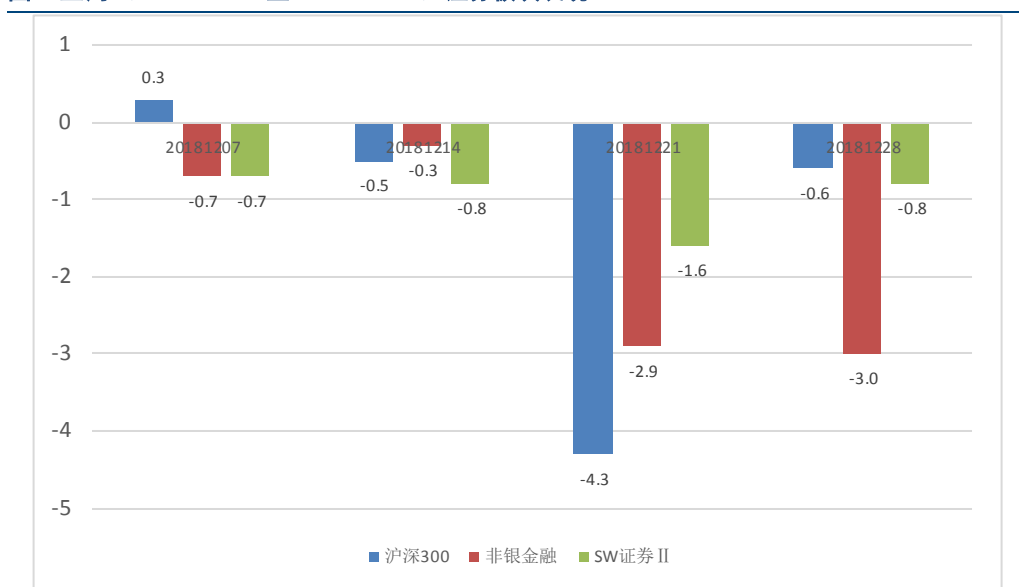
图1:上周(2018-12-24至2018-12-28)证券板块表现
