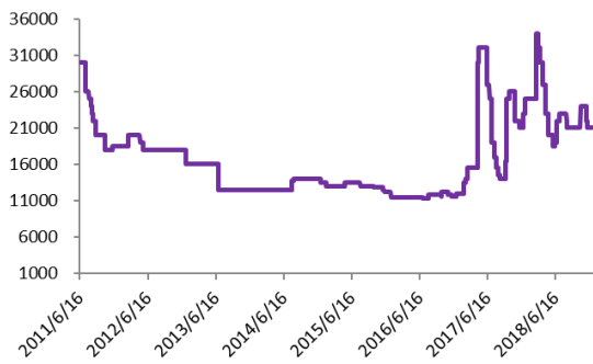
图表43: R32 价格走势 (元/吨)
