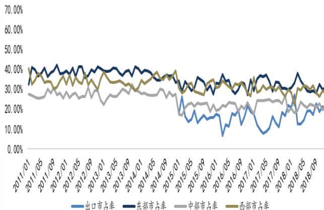
图 20: 国内东中部市占率上升, 出口销量同比-7%
