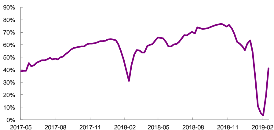
图 7：全国 53 座电弧炉产能利用率（周度，截至 2019/3/1）
