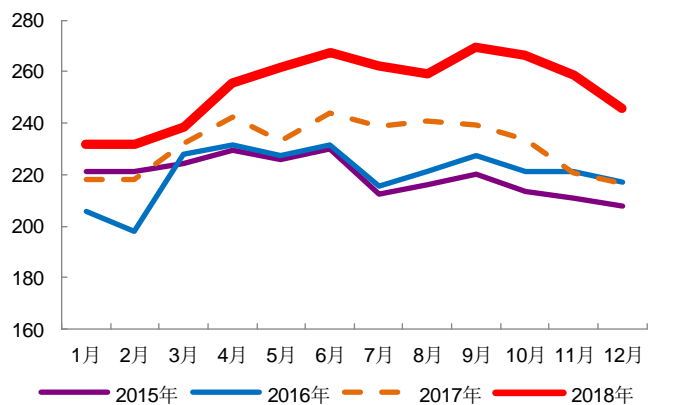
图 3：全国粗钢月度日均产量（万吨，2018 年 12 月）
