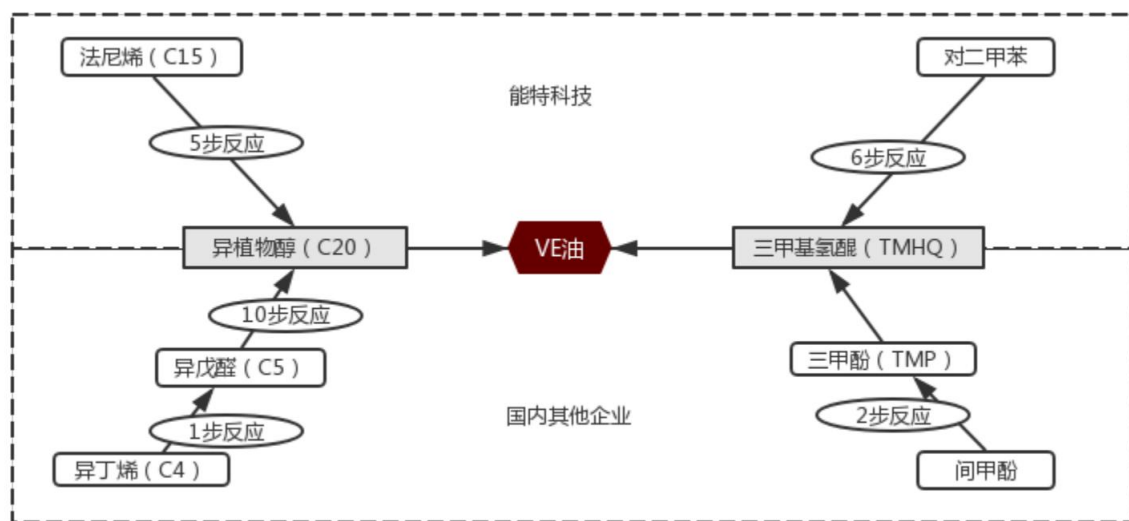
图表 1：VE 合成工艺路线图
