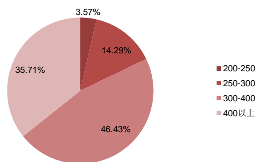
图 2：2019 年第 2 批推广目录乘用车续航里程统计
