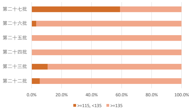
图 3: 近 6 批推广目录客车能量密度统计
