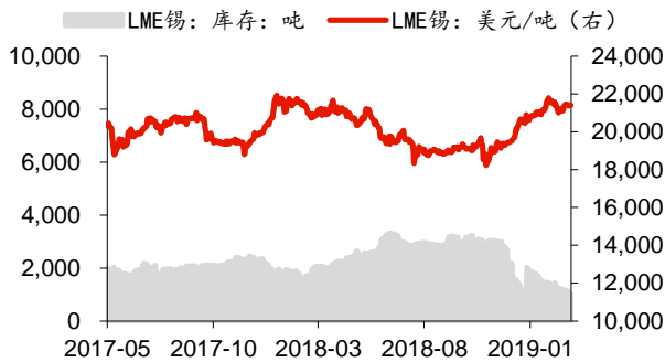
图表18: LME 期货锡价及库存
