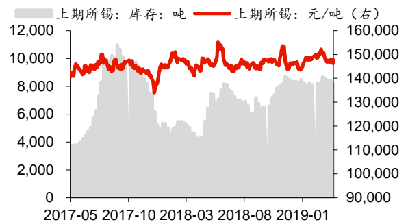
图表19: SHFE 期货锡价及库存
