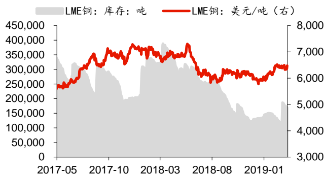
图表8：LME 期货铜价及库存
