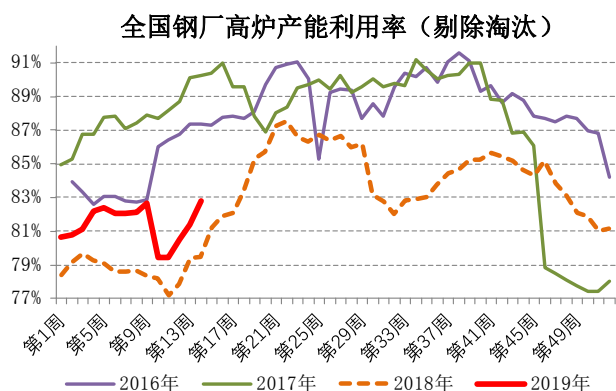
图 7: Mysteel 全国 163 家钢厂高炉产能利用率
