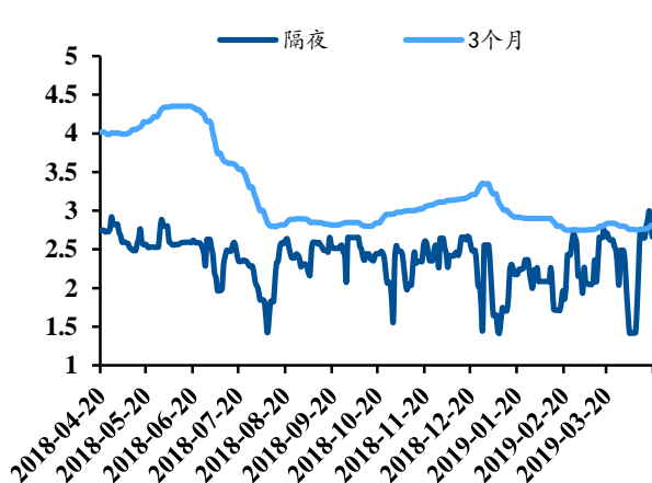
图 28: SHIBOR (%)
