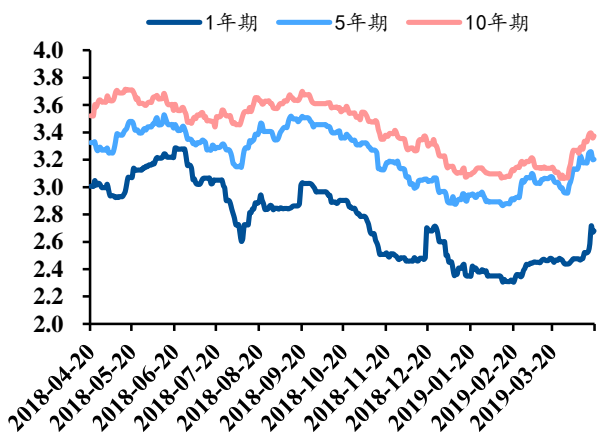
图 27: LIBOR (%)
