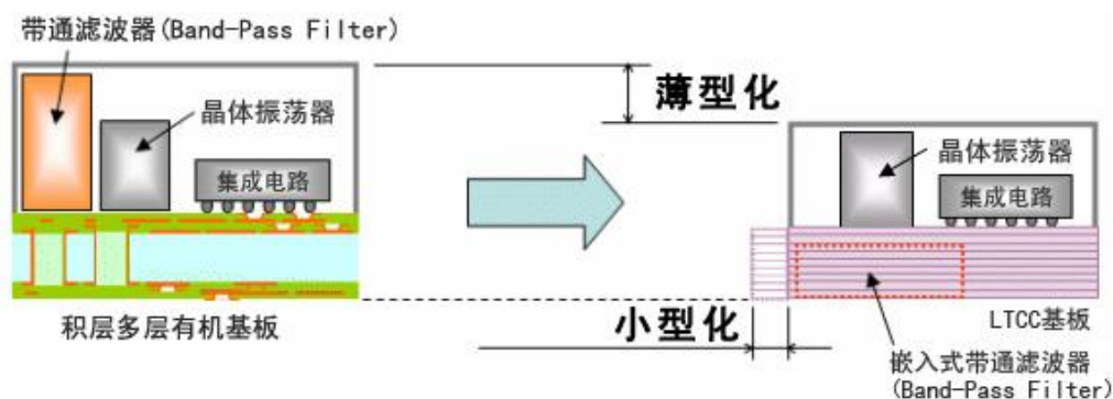
图表12： 京瓷对安装于基板上的带通滤波器、平衡/不平衡转换器等元件进行嵌入化设计的方案示意图
