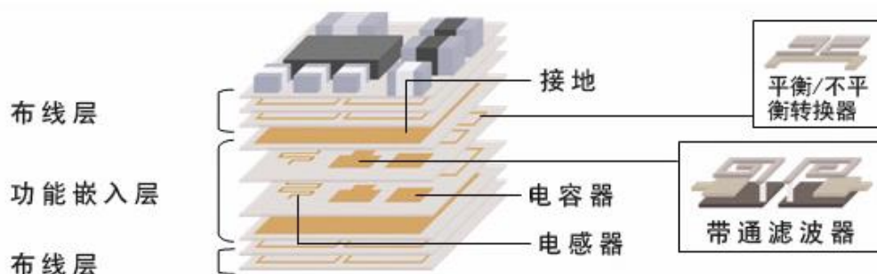
图表6: LTCC 产品结构图
