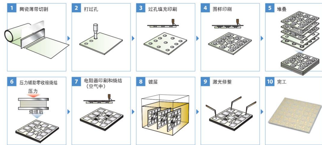
图表5：LTCC 工艺流程
