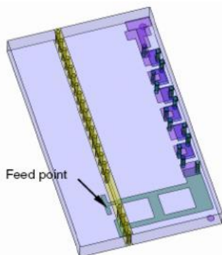
图表13： 蓝牙模块的 LTCC 倒 F 天线示意图
