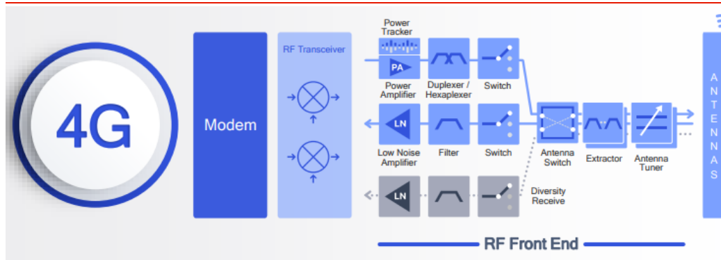
图表11： 4G 终端的射频前端结构图
