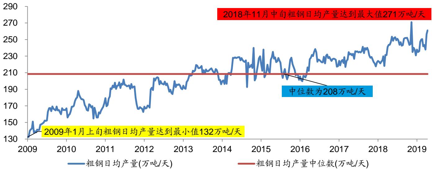
图 7：2009年1月至今全国预估粗钢旬日均产量
