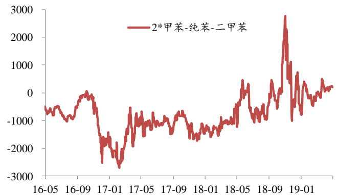
图表 11: 2*甲苯-纯苯-二甲苯
