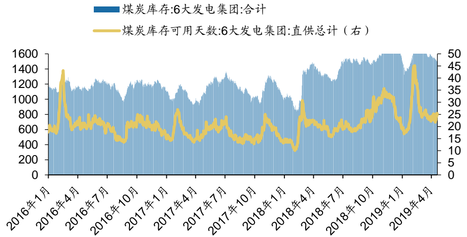
图32：六大发电集团煤炭库存（万吨）
