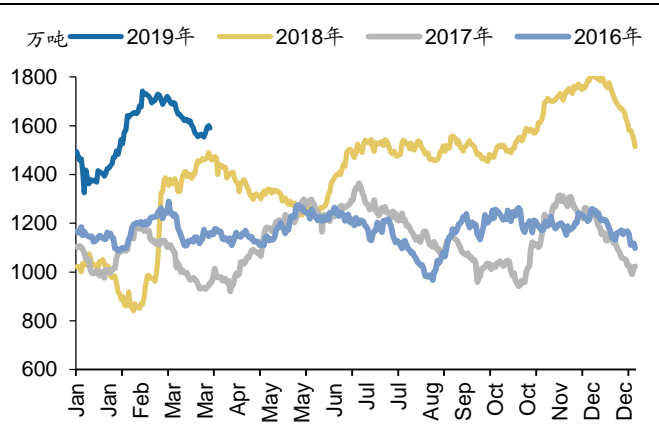
图36: 六大电厂电煤库存量(万吨)
