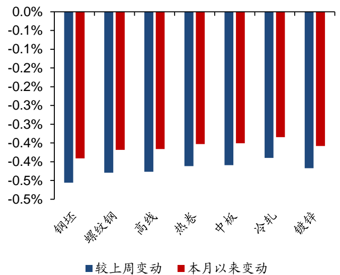
图 16: 分品种钢材短流程成本变化
