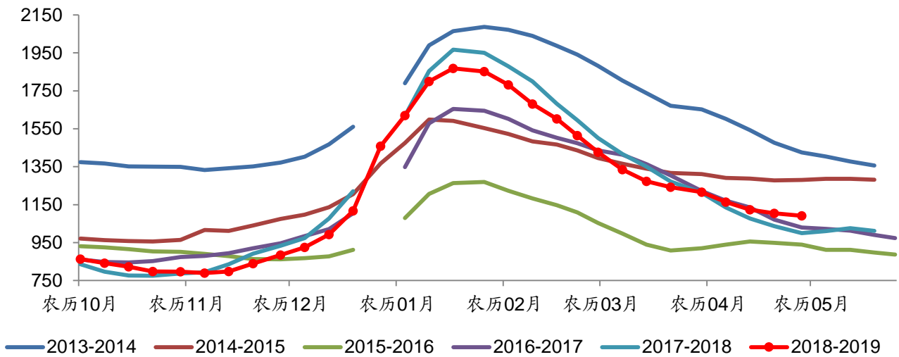
图 9: 2013年至今钢材周度社会库存(单位: 万吨, 农历日历坐标轴)
