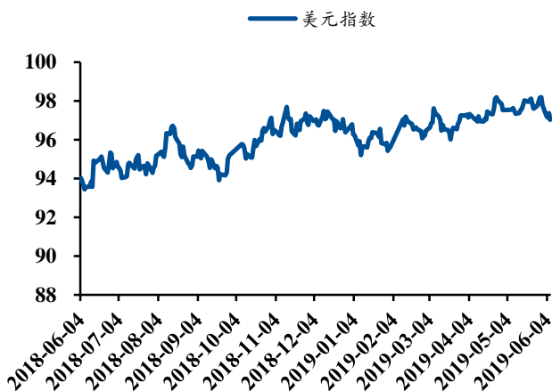
图 21：美元指数
