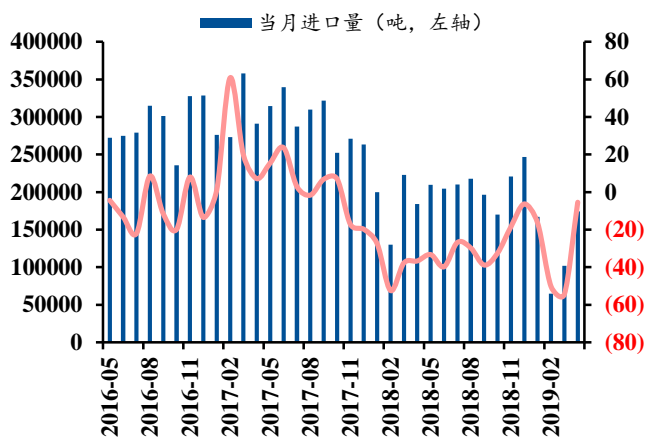
图 41: 废铜进口量
