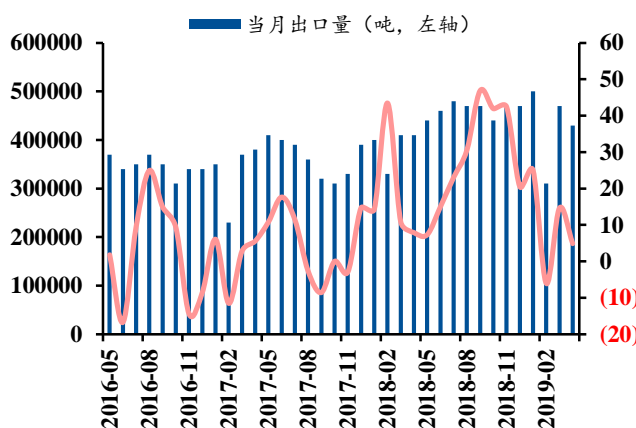
图 46: 铝材出口量
