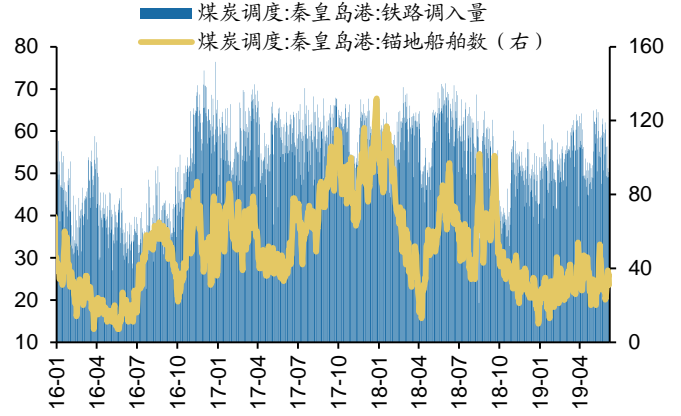
图32: 秦皇岛煤炭调入量(万吨)/锚地船舶(艘)
