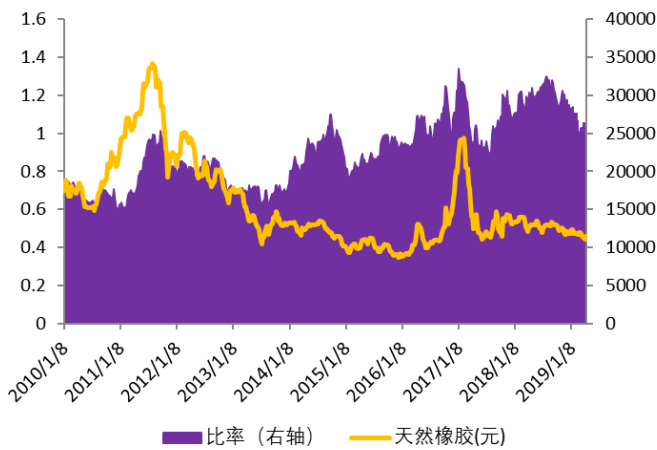
图表81: 丁苯/天胶比率走势
