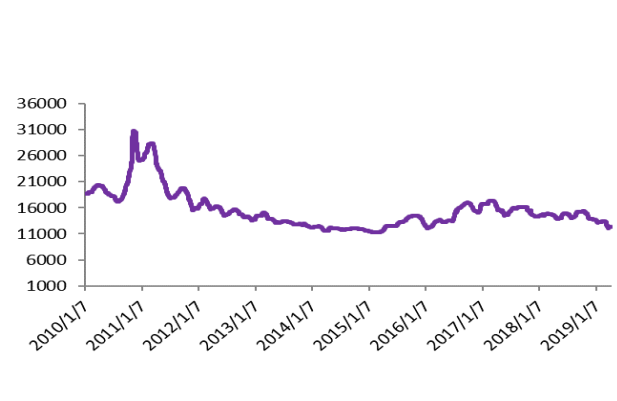
图66: 粘胶短纤价格走势 (元/吨)
