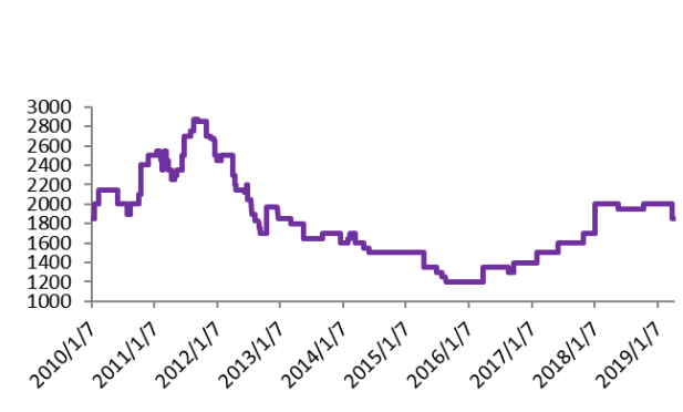
图表92: 硝酸铵 (工业) 价格走势 (元/吨)
