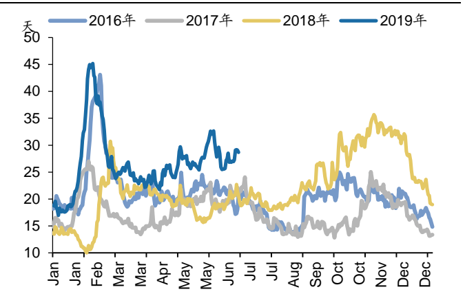
图42: 六大电厂电煤库存可用天数(天)
