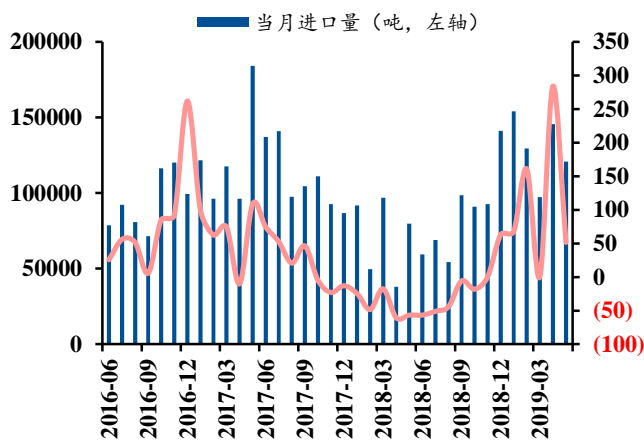
图 52: 镍铁进口量
