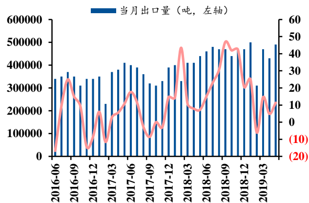
图 46: 铝材出口量
