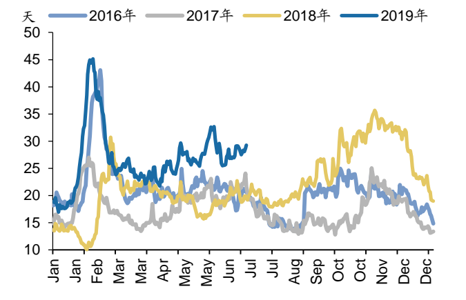
图44: 六大电厂电煤库存可用天数(天)
