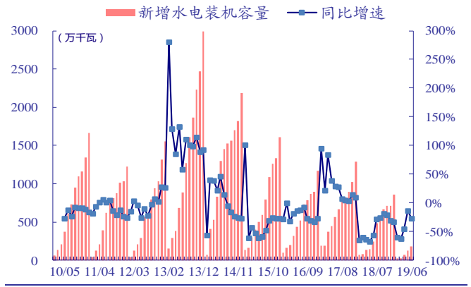
图 19: 新增水电装机容量及同比变化
