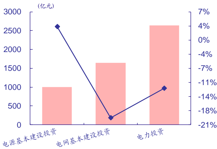
图 13: 2019 年 6 月电力投资累计完成额
