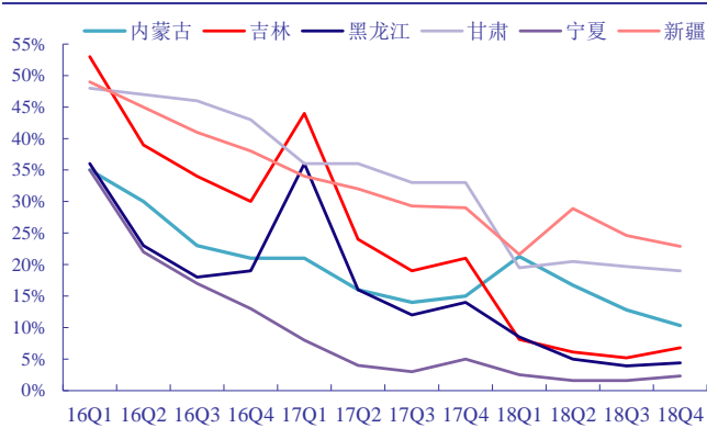
图 23: 6 大主要地区弃风率
