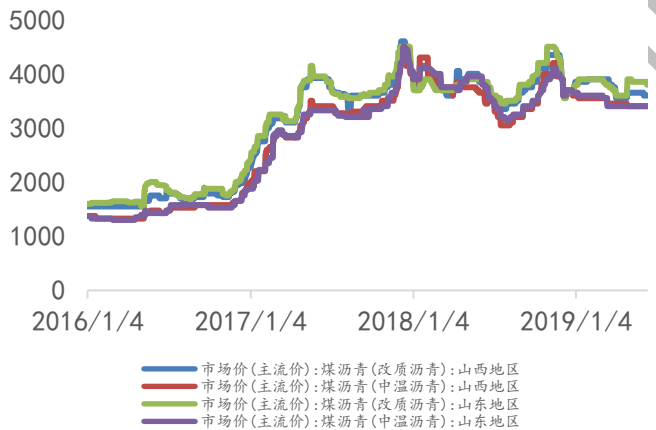
图表 21. 煤沥青价格走势(元/吨)
