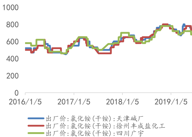
图表 17. 氯化铵价格走势(元/吨)
