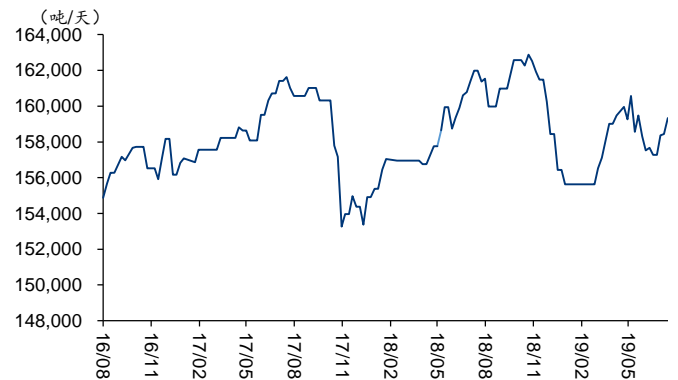
图表65: 全国浮法玻璃日熔量
