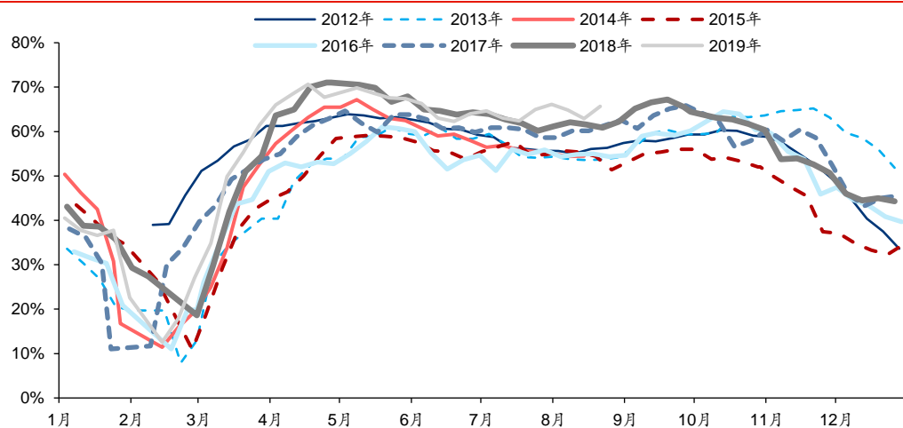
图表53: 2012-2019年全国磨机月度开工率比较
