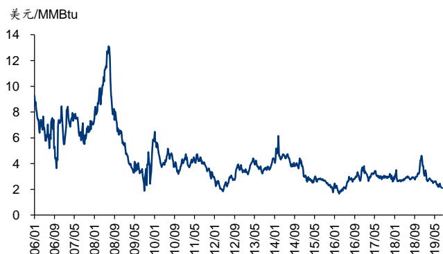
图表122: 美国 HenryHub 天然气现货价格走势
