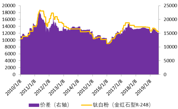
图表103: 钛白粉金红石型价格价差(元/吨)
