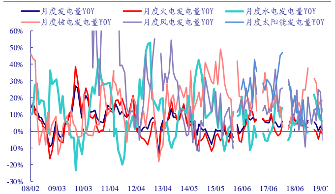
图 5: 月度发电量及增速
