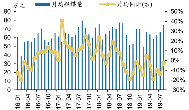
图39: 六大电厂月度日均耗煤量 (万吨)
