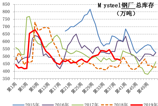
图 10: Mysteel 钢厂钢材总库存 (万吨)
