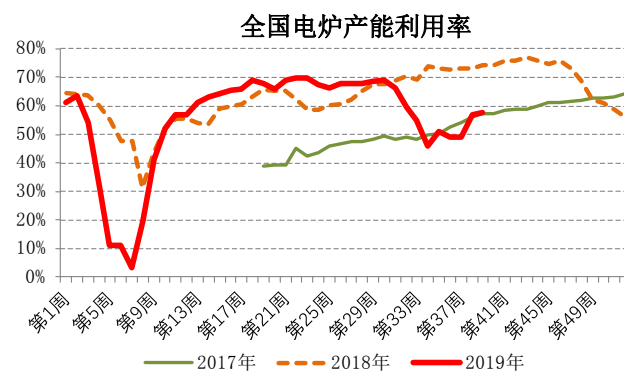
图 8：Mysteel 全国 53 家电炉钢厂产能利用率
