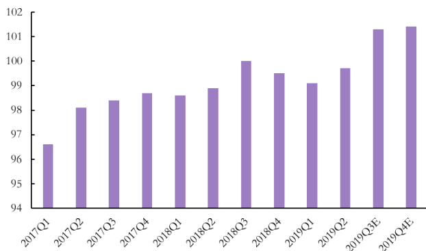
图 18: 全球石油需求及预测 (百万桶/天)
