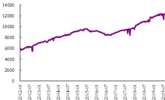
图 29: 美国原油产量 (千桶/天)
