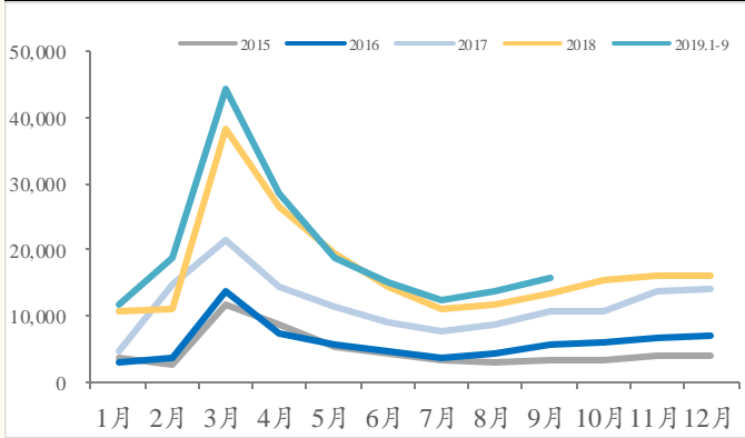
图表 9：挖掘机行业销量：1-9 月同比增长 14.7%
