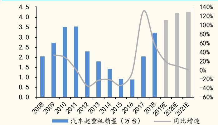
图表 8：预测 2019-2021 年汽车起重机复合增速 10%
