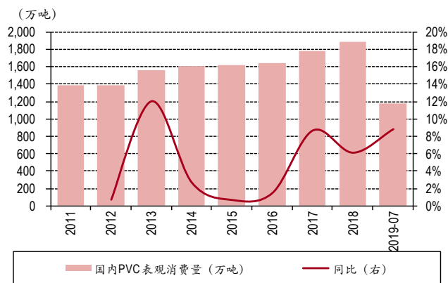
图表 29.历年 PVC 表观消费量
