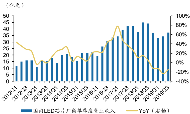
图44: 中国大陆主要LED芯片企业单季度营收趋势
