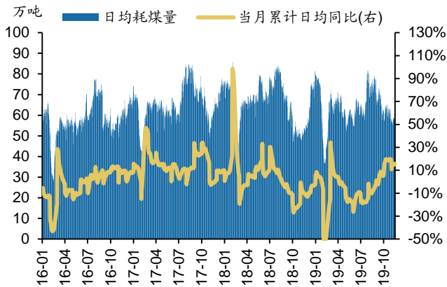
图40: 六大电厂日均耗煤量(万吨)
