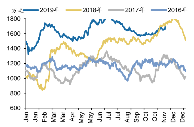
图38: 六大电厂电煤库存量(万吨)
