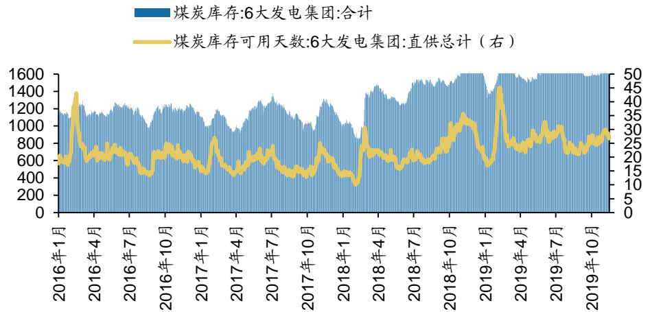
图34：六大发电集团煤炭库存（万吨）
